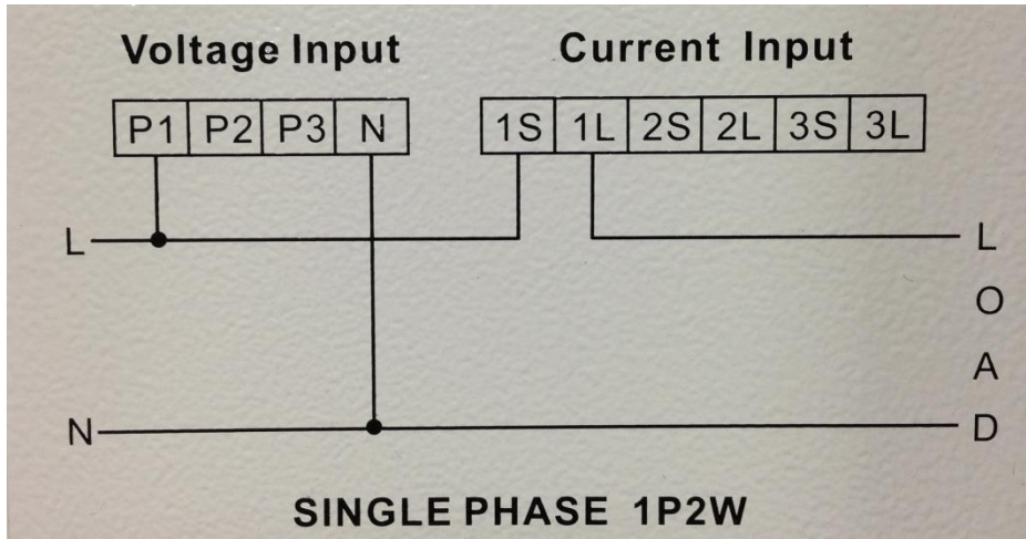
接線圖
